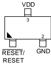
SOT-23-3
