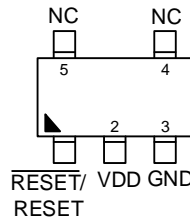
SOT-23-5
