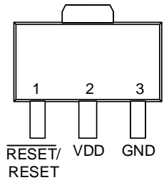
SOT-89
