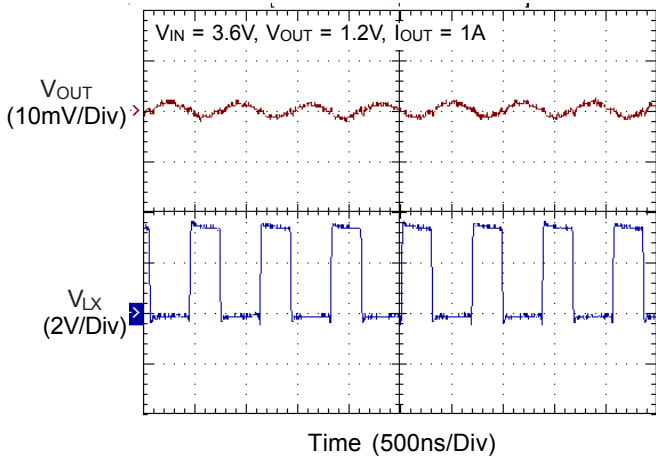
Ripple
