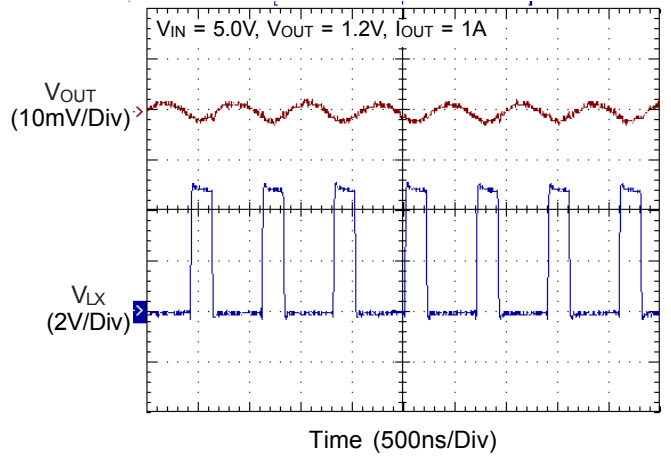
Ripple
